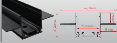
Siva Altı Alüminyum Ray Recessed Aluminum Track
