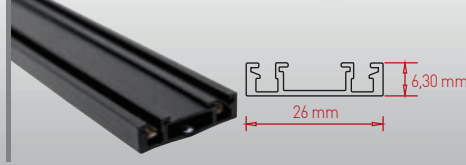
Siva Üstü Alüminyum Ray Surface Aluminum Track
